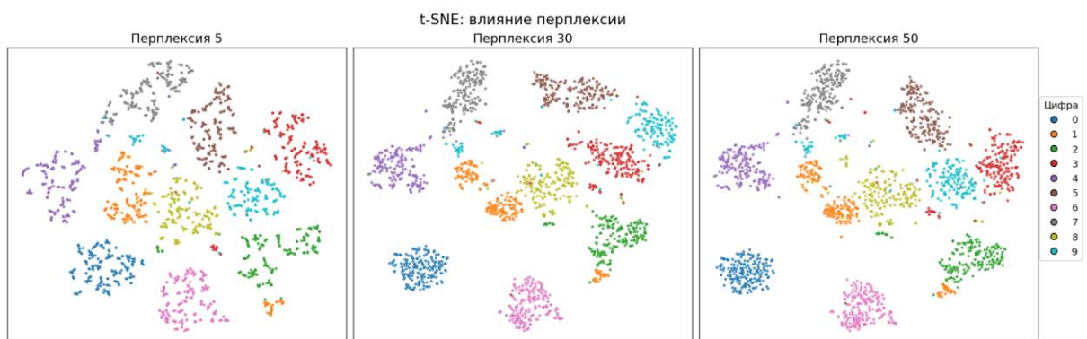
Рисунок 4 – Проекции t-SNE для трёх значений перплексии
